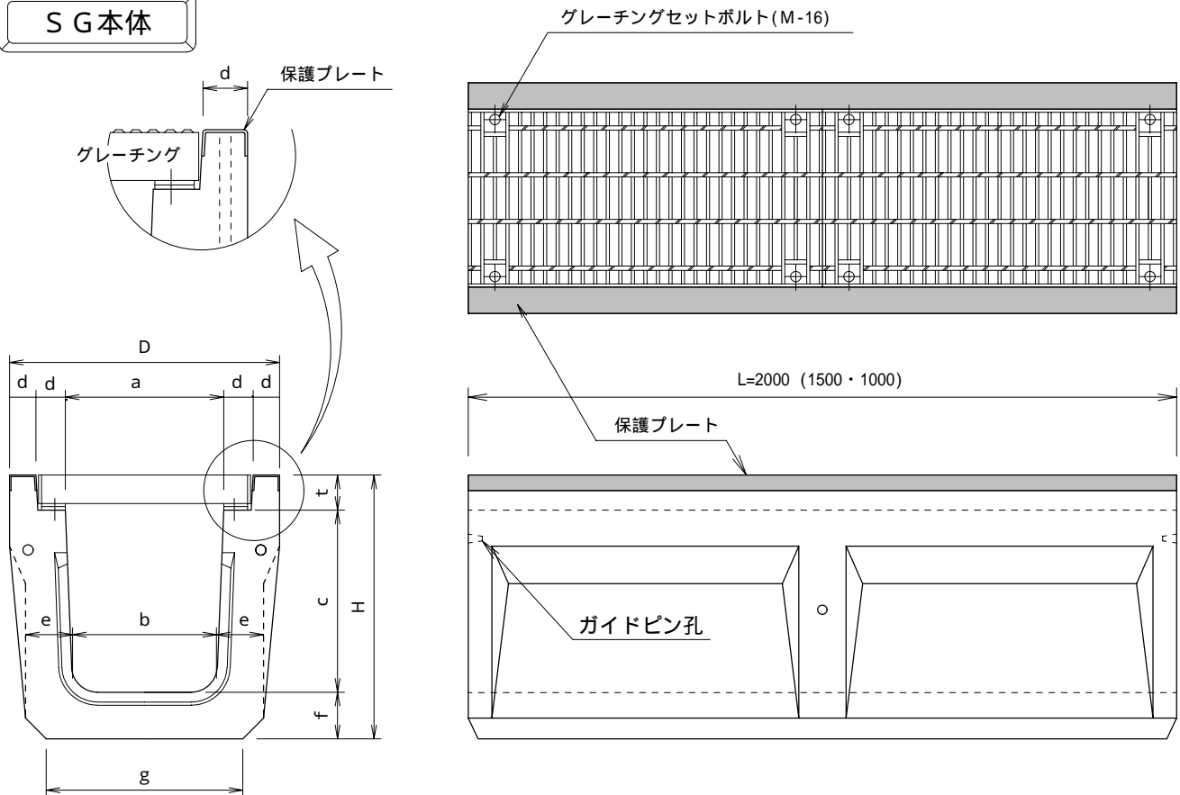
横断用S G側溝<グレーチング型・保護プレート付き> 寸法表
