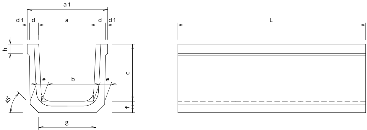
道路用側溝：寸法重量表
